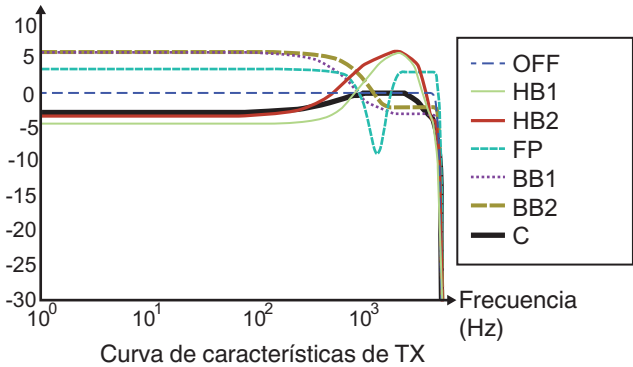
Curva de características de TX
