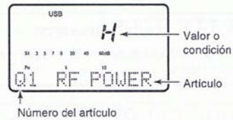
[EJEMPLO DE PANTALLA: MODO DE AJUSTE RÁPIDO]
